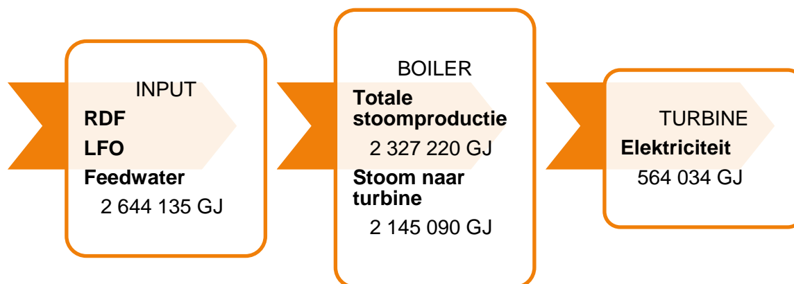
Figuur 2: Energiestromen 2022
